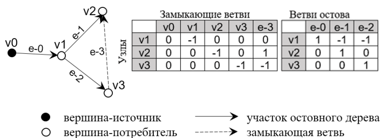
Рис. 1. К построению матрицы соединений кольцевой газовой сети
